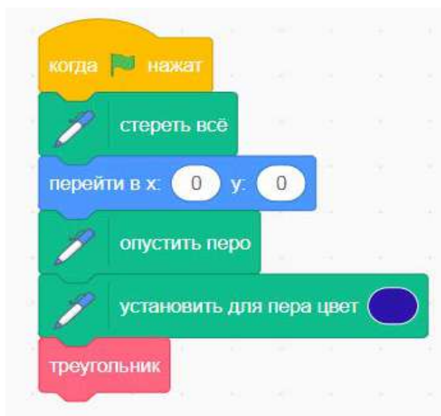
Рис. 137. Вид программы с новым блоком
